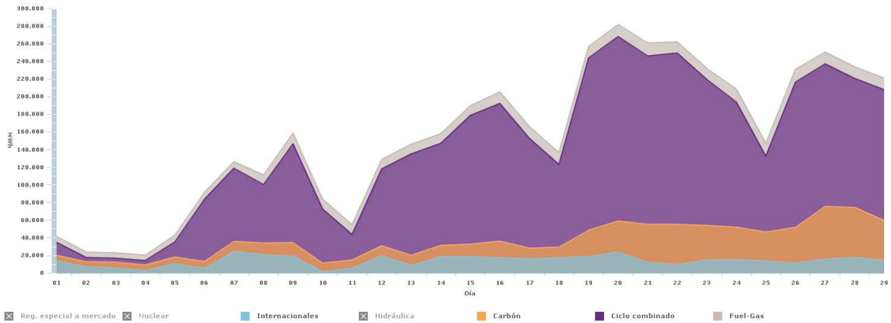
04/2010 - Energía diaria por tecnologías - País: Mibel
